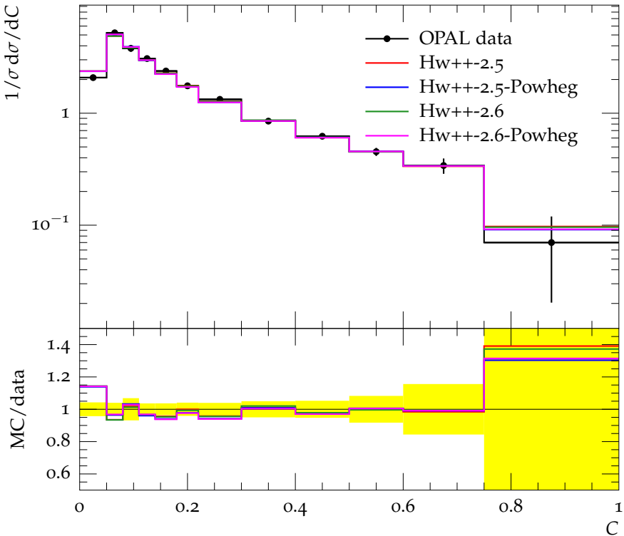
C parameter at 197 (189–209) GeV
