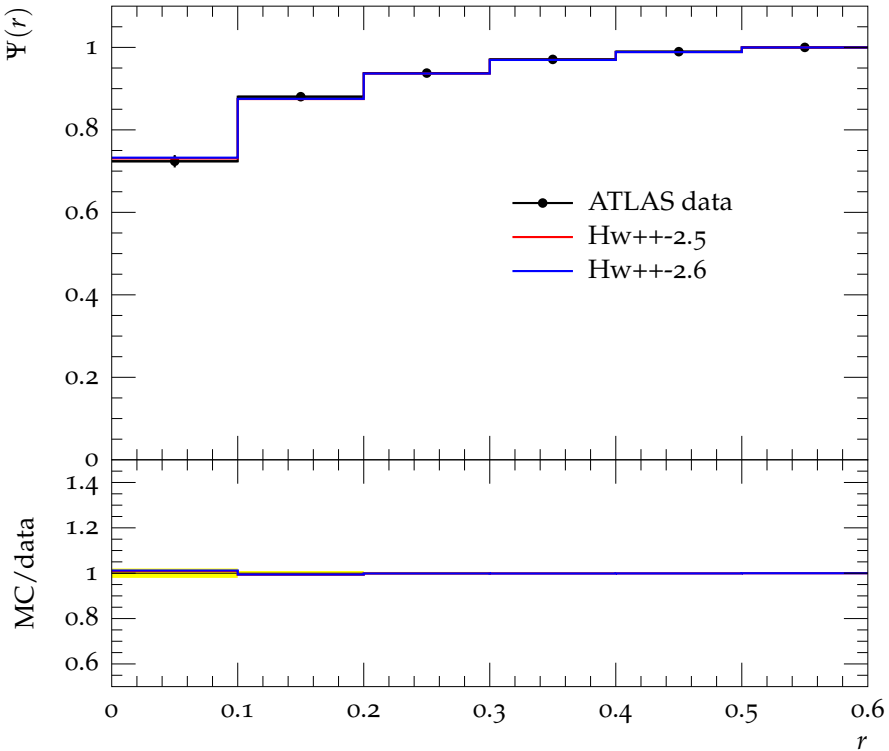
Jet shape \Psi for p_{\perp} \in 310\text{--}400\text{ GeV} , y \in 0.3\text{--}0.8
