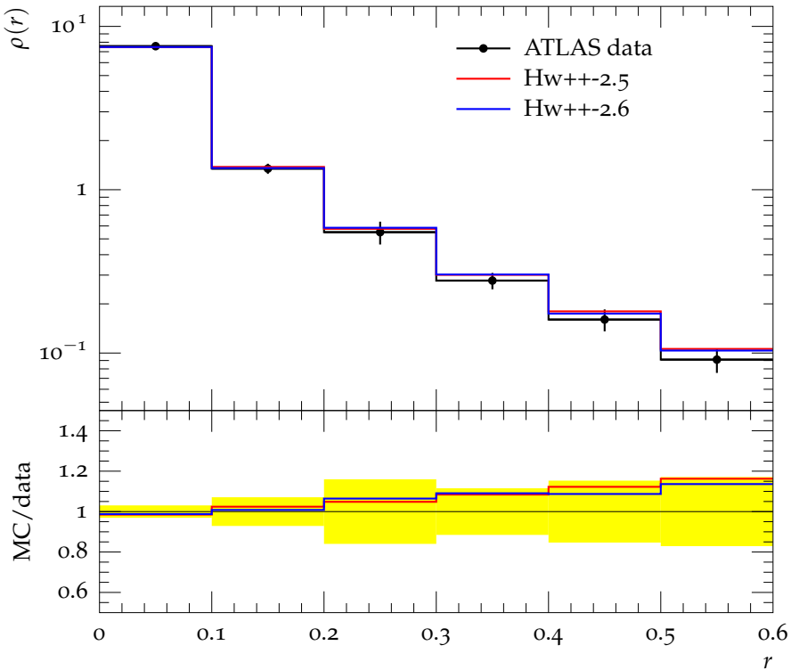
Jet shape \rho for p_{\perp} \in 310\text{--}400\text{ GeV} , y \in 0.8\text{--}1.2
