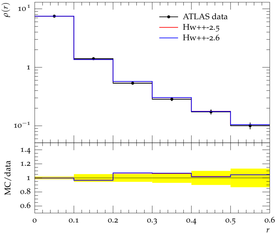
Jet shape \rho for p_{\perp} \in 310\text{--}400\text{ GeV} , y \in 0.0\text{--}2.8
