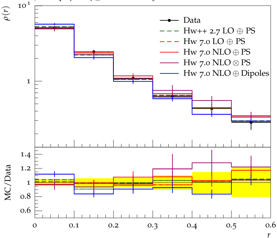
Jet shape \rho for p_{\perp} \in 60\text{--}80\text{GeV} , y \in 0.8\text{--}1.2
