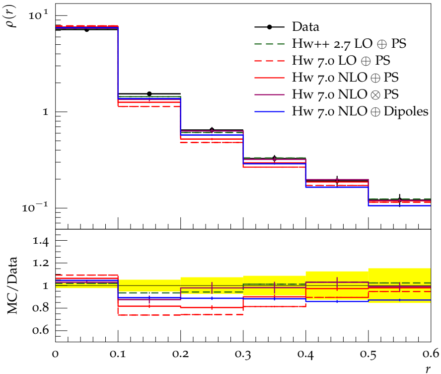
Jet shape \rho for p_{\perp} \in 260\text{--}310\text{ GeV} , y \in 0.8\text{--}1.2
