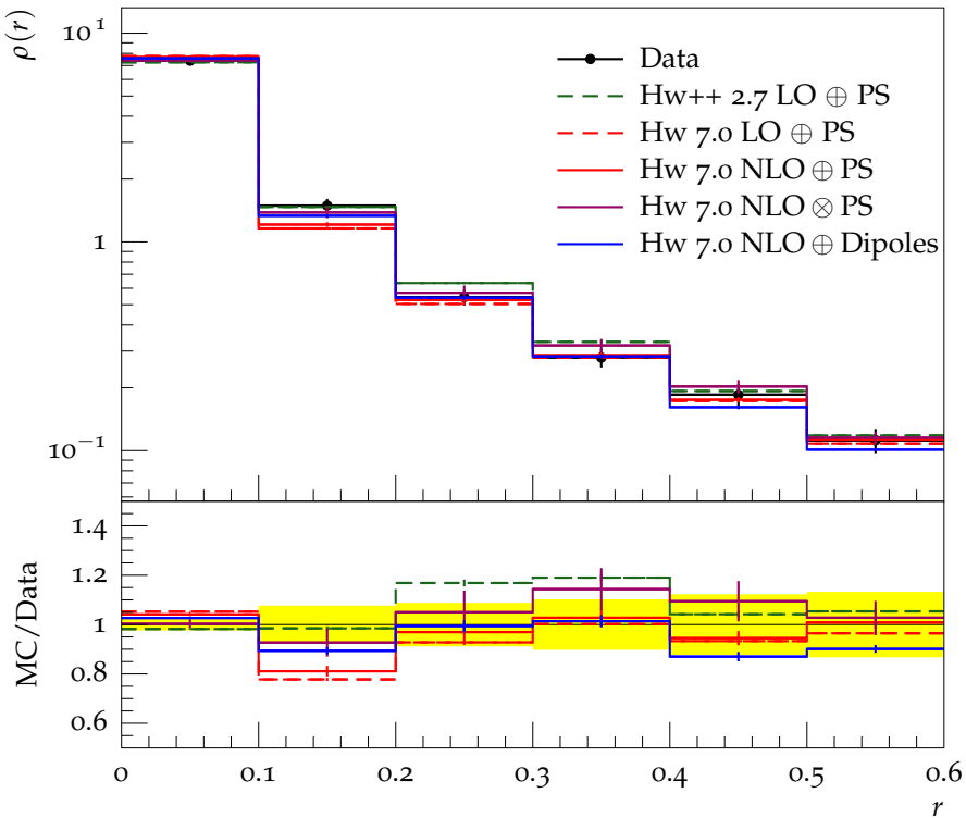
Jet shape \rho for p_{\perp} \in 310\text{--}400\text{ GeV} , y \in 0.0\text{--}0.3
