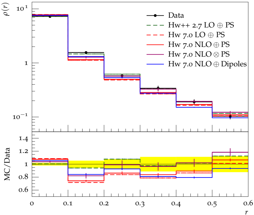
Jet shape \rho for p_{\perp} \in 310\text{--}400\text{ GeV} , y \in 0.3\text{--}0.8
