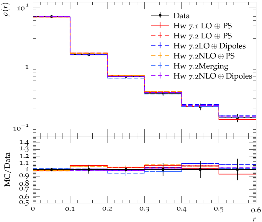
Jet shape \rho for p_{\perp} \in 210\text{--}260\text{ GeV} , y \in 0.8\text{--}1.2
