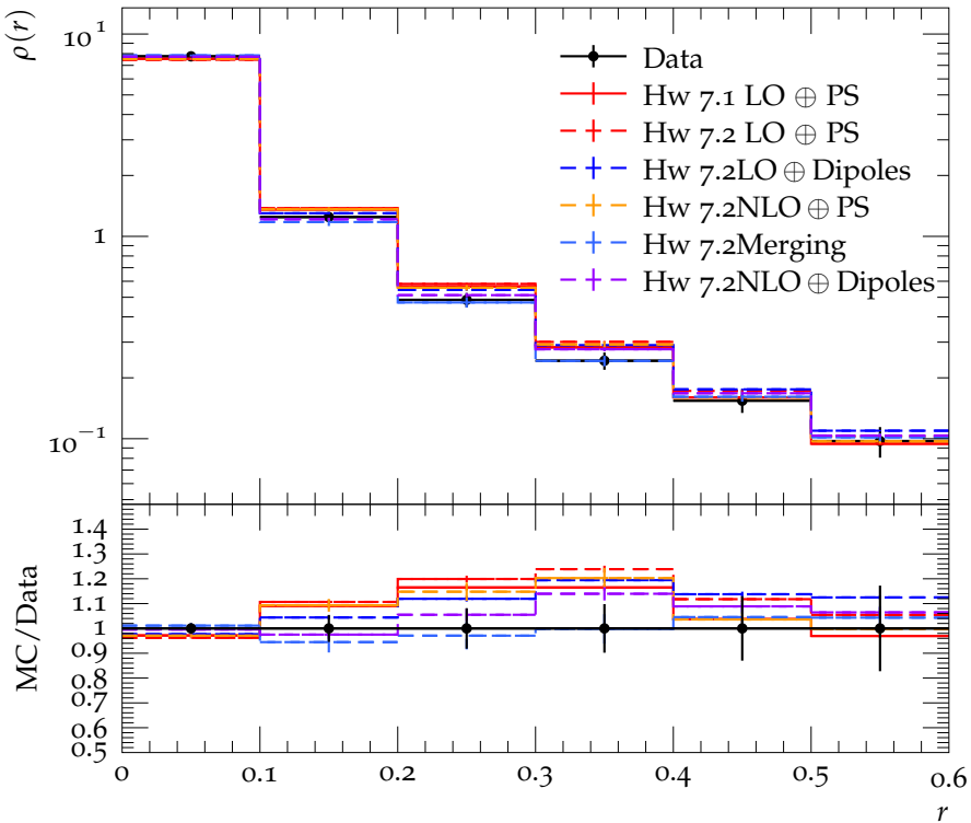
Jet shape \rho for p_{\perp} \in 310\text{--}400\text{ GeV} , y \in 1.2\text{--}2.1
