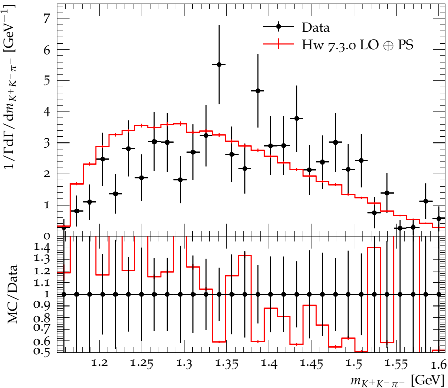
K^+K^-\pi^- mass distribution in D_s^+ \rightarrow K^+K^-\pi^+\pi^-\pi^-
