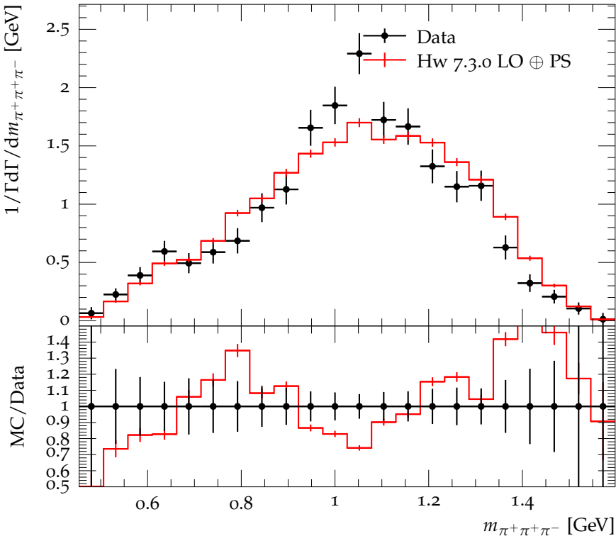
\pi^+\pi^+\pi^- mass distribution in D^0 \rightarrow 2\pi^+2\pi^-\pi^0
