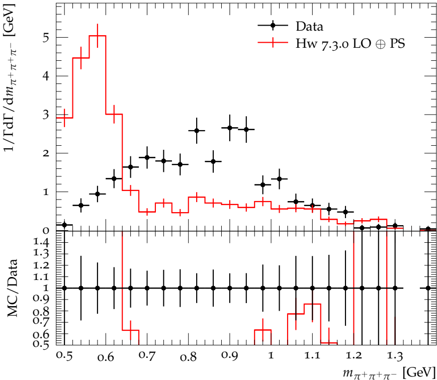
\pi^+\pi^+\pi^- mass distribution in D^0 \rightarrow 2\pi^+2\pi^-2\pi^0
