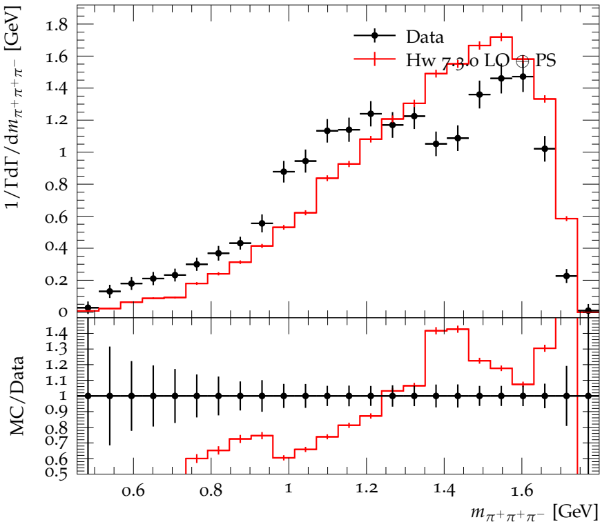
\pi^+\pi^+\pi^- mass distribution in D^+ \rightarrow 2\pi^+\pi^-\pi^0
