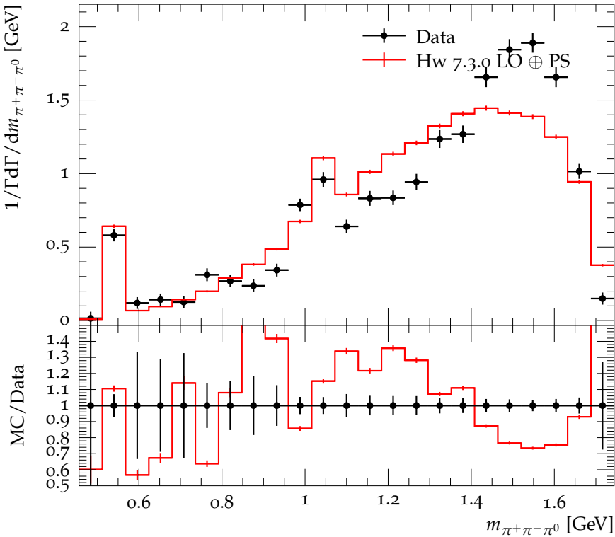
\pi^+\pi^-\pi^0 mass distribution in D^+ \rightarrow 2\pi^+\pi^-\pi^0
