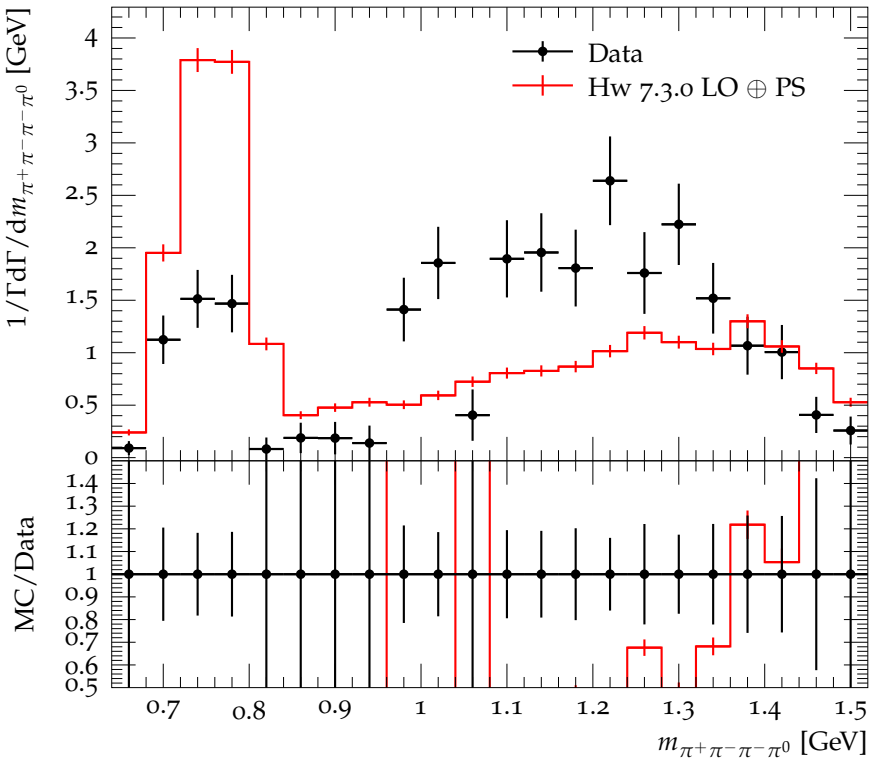
\pi^+\pi^-\pi^-\pi^0 mass distribution in D^+ \rightarrow 3\pi^- + 2\pi^-\pi^0
