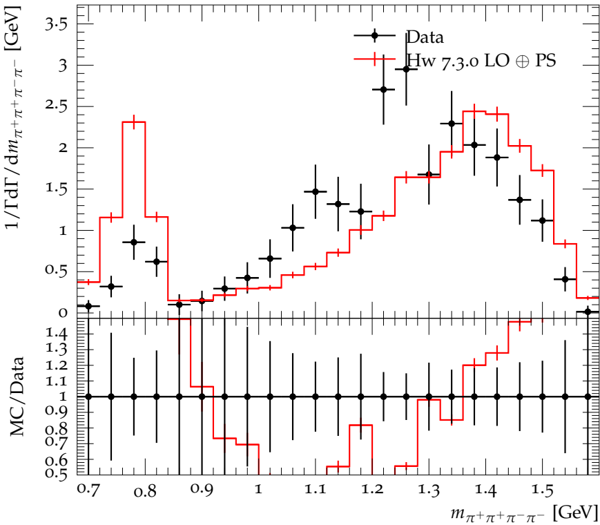
\pi^+\pi^+\pi^-\pi^- mass distribution in D^+ \rightarrow 3\pi^+2\pi^-\pi^0
