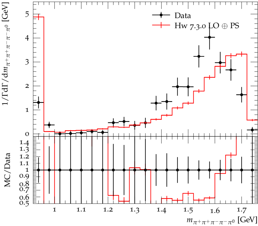
\pi^+\pi^+\pi^-\pi^-\pi^0 mass distribution in D^+ \rightarrow 3\pi^+2\pi^-\pi^0
