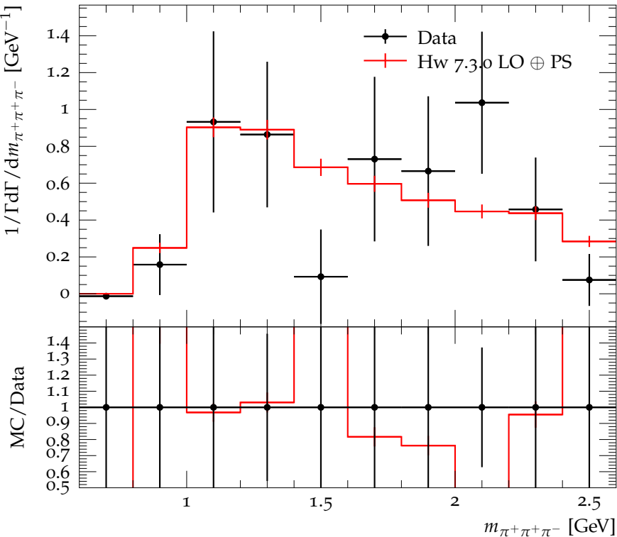
\pi^+\pi^+\pi^- mass distribution in B_c^+ \rightarrow \psi(2S)\pi^+\pi^+\pi^-
