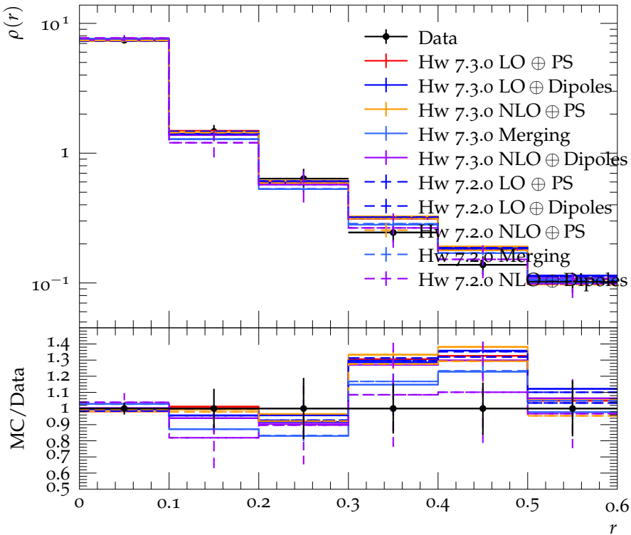
Jet shape \rho for p_{\perp} \in 400\text{--}500\text{ GeV} , y \in 0.0\text{--}0.3
