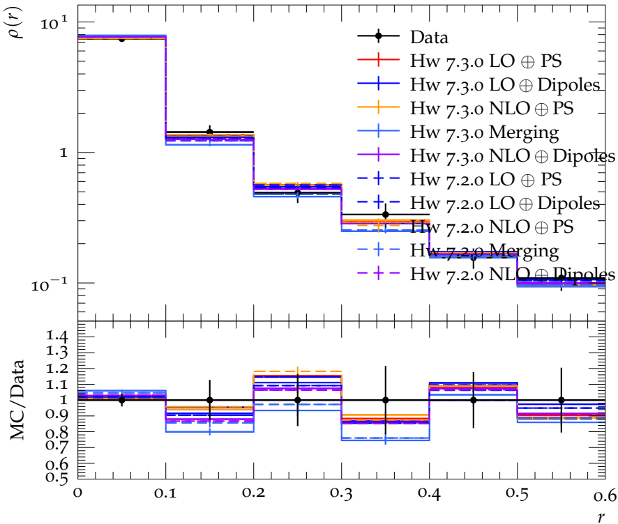
Jet shape \rho for p_{\perp} \in 400\text{--}500 GeV, y \in 0.8\text{--}1.2
