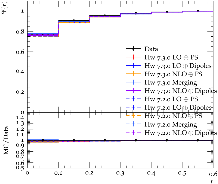
Jet shape \Psi for p_{\perp} \in 400\text{--}500\text{ GeV} , y \in 0.0\text{--}2.8
