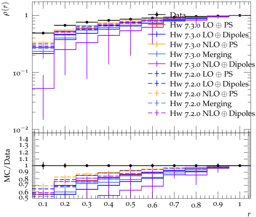
Jet shape \rho for p_{\perp} \in 45\text{--}70\text{ GeV} , \eta \in 2.5\text{--}3.5
